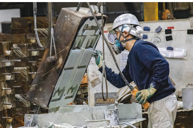
押し固めた砂型にコーティング剤を塗り、細かいところを調整
