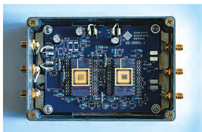
ダイヤモンドデバイス信号増幅回路
