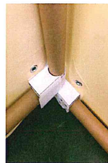
紙管接合部：マジックテープで固定
