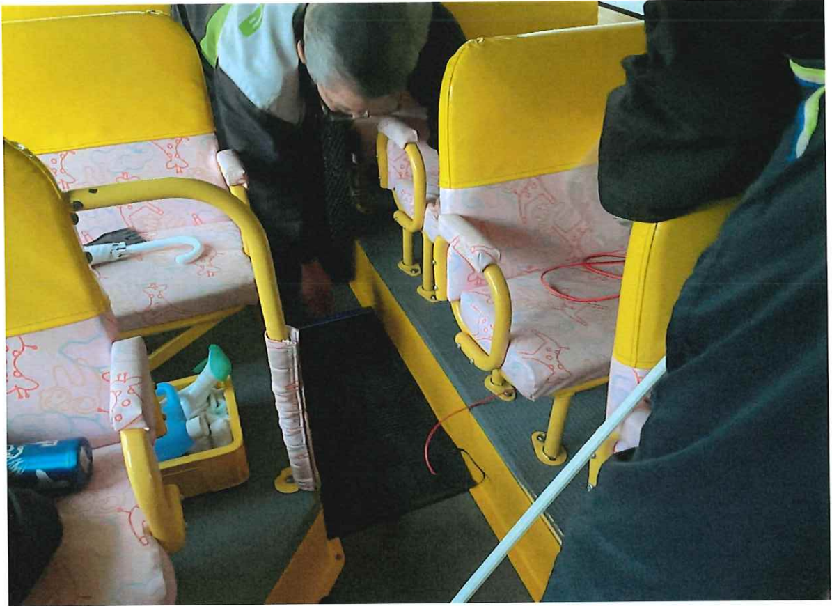
通路に感圧マットを取付
